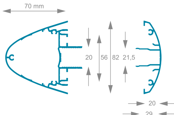
PYLON 50R
