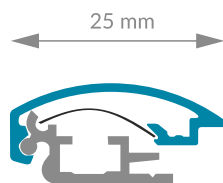
PROFIL OWZ 25 mm
