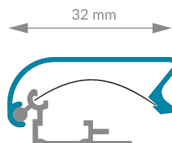
PROFIL OWZ 32 mm
