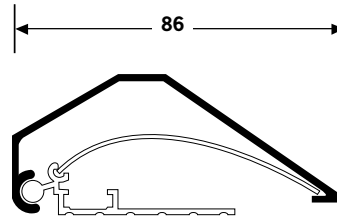
139160 Display klemprofil 86 Display clamping springs 86 Display klemprofil 86
