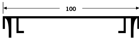
137200 Display lichtbakprofil Display LightBoxprofile Display lichtkastprofil
